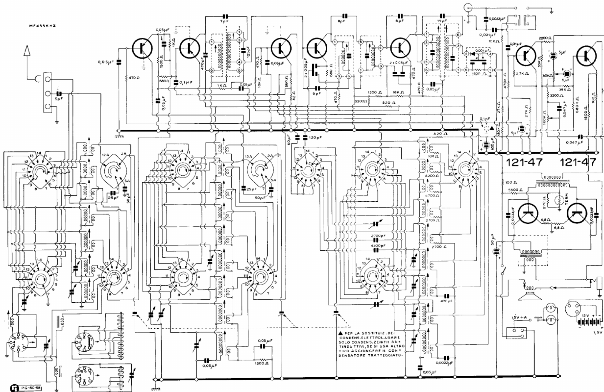
Fig. 2 - Lo schema elettrico del radiorecettore Zenith mod. Royal 1000 D.
